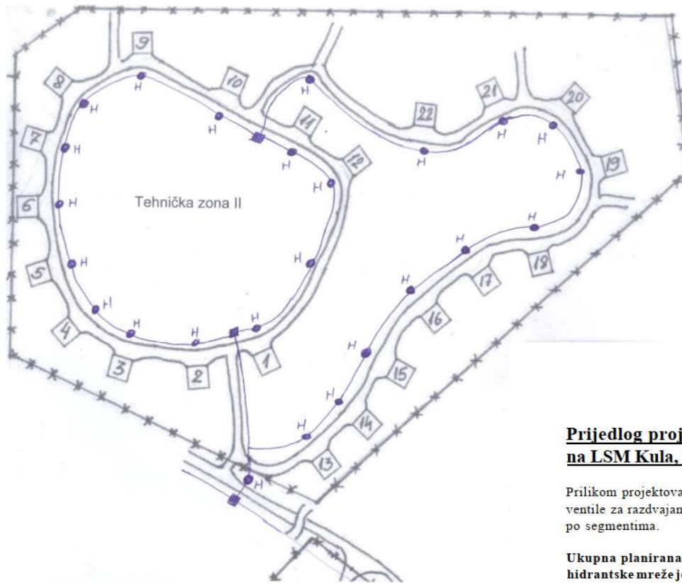
SL.2 Šema skladišta Kula sa hidrantskom mrežom
